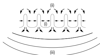
(i). ダイアフラムの動き (ii). 発生する気流の方向 (iii). 気流が発生させるアコースティック・ウェーブ
